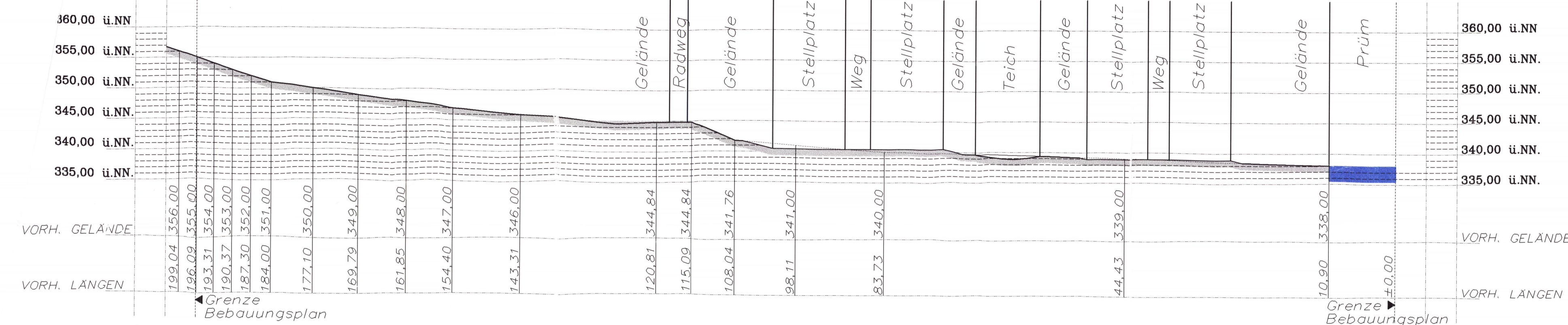
QUERSCHNITT I-I, M=1:500
