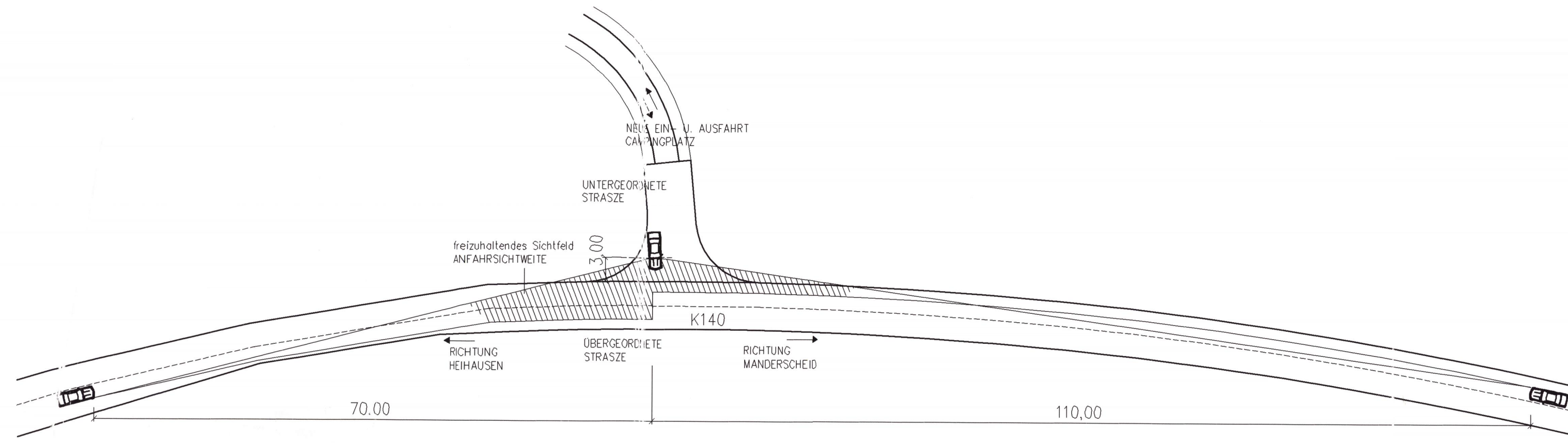
SICHTFELD, M=1:500
