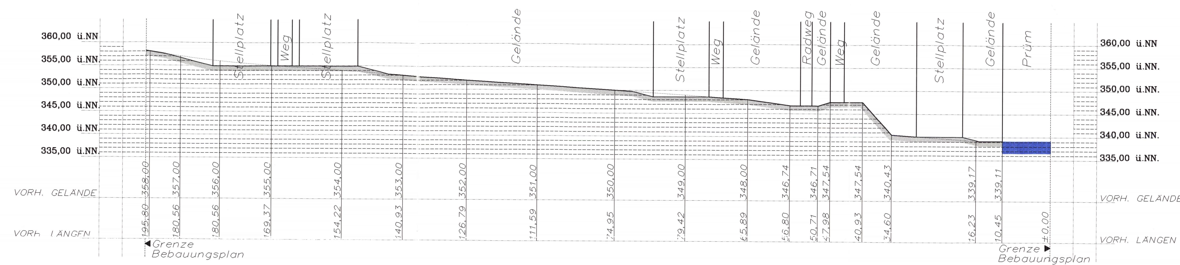
QUERSCHNITT II-II, M=1:500
